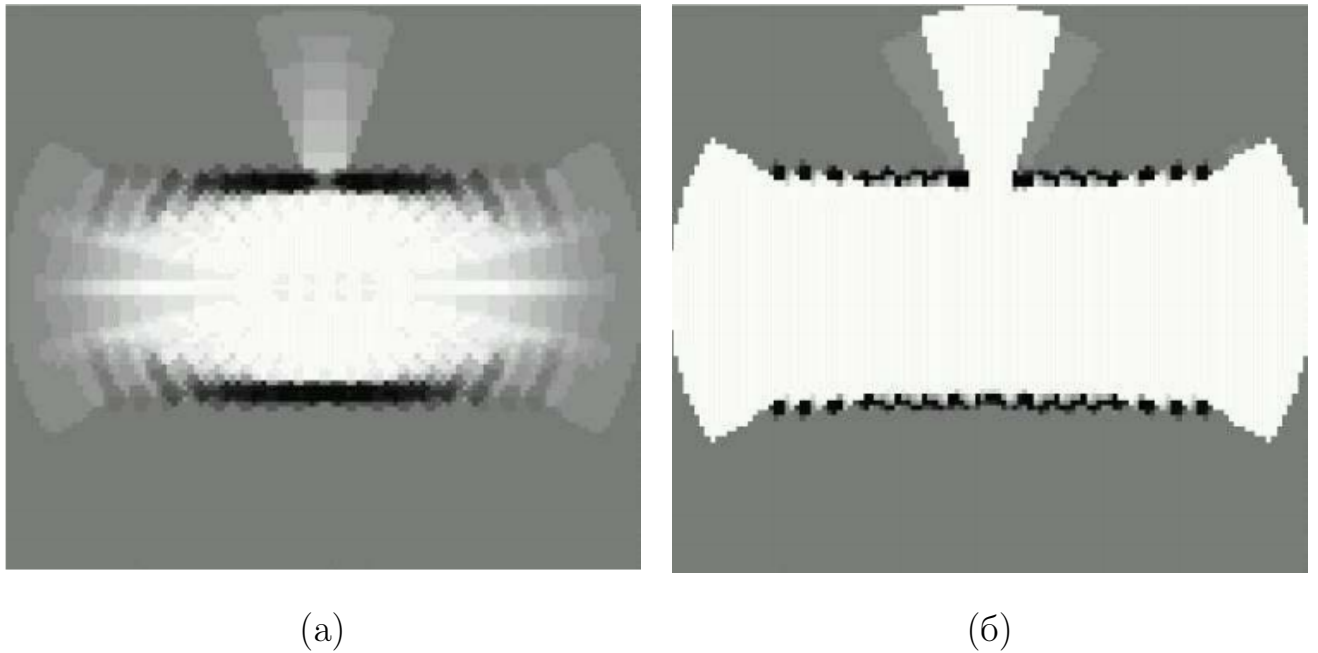
Рис. 1.2. Результаты картирования двери из работы [7]. (а) - результаты алгоритма на основе обратной модели, (б) - на основе EM-алгоритма с прямой моделью.
